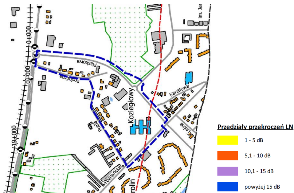
Mapa terenów zagrożonych hałasem dla odcinka drogi wojewódzkiej nr 196 - wskaźnik L_N [dB] Źródło: https://www.wzdw.pl/
