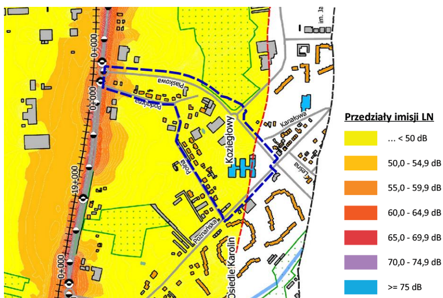
Mapa imisyjna dla odcinka drogi wojewódzkiej nr 196 - wskaźnik L_N [dB] Źródło: https://www.wzdw.pl/
