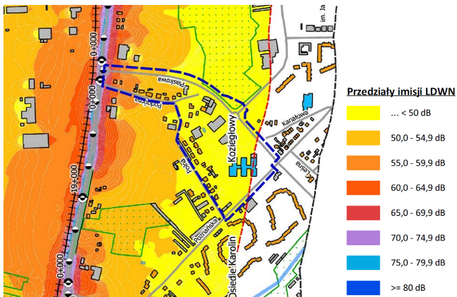
Mapa imisyjna dla odcinka drogi wojewódzkiej nr 196 - wskaźnik L_{DWN} [dB] Źródło: https://www.wzdw.pl/
